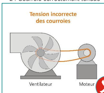
3 : Schémas de courroie non tendue
