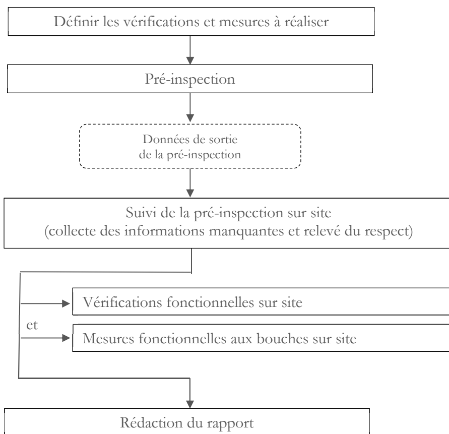
Figure 1 : Organisation générale d'un diagnostic d'une installation de ventilation RE2020
