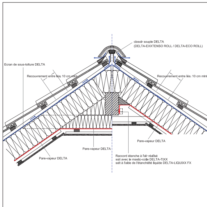
Détail en faîtage.
