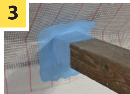
Après (pare-vapeur DELTA®-REFLEX, bande adhésive DELTA®-MULTI-BAND et étanchéité liquide DELTA®-LIQUIXX FX)
