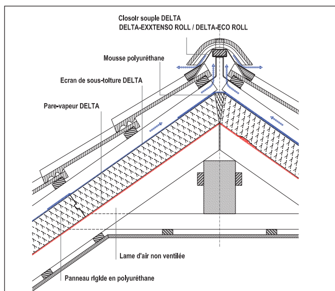
Détail en faîtage.
